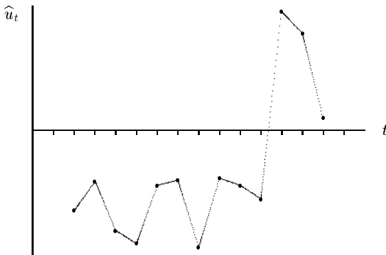
図 4：正の系列相関
